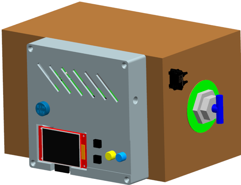
Infraschall-Messgerät: Druckkörper (braun) mit montiertem 3D-Druck-Gehäuse (grau) mit eingelassenem Display (rot). Grafik: privat
